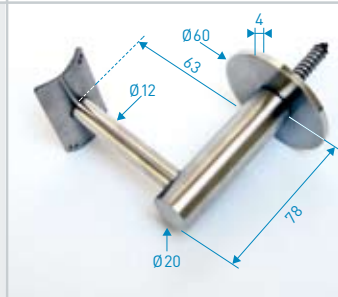
Wandhalterung Nr. 042 • 33,7 / 42,4 mm • € 18,20
