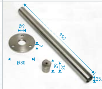
Brüstungsteil 3-teilig Nr. 030 • 33,7 / 42,4 mm • € 26,10
