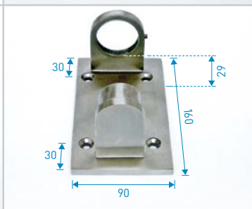
Pfostenhalter Nr. 101 • 42,4 mm • € 48,30
