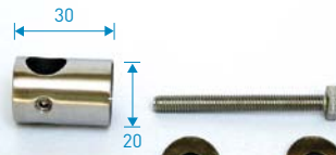
Glshalter Nr. 269W • f. 8-12,76 mm Glas € 13,20
