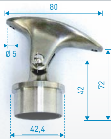
Gelenkstück Nr. 240 • 42,4 mm • € 17,80
