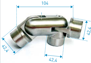
3-Wege Gelenk f. Rohr Nr. 251 • 42,4 mm • € 40,10
