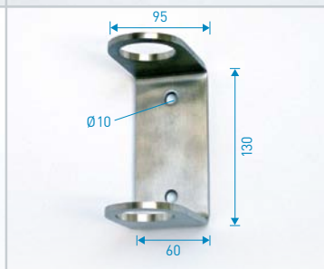
Pfostenhalter klein Nr. 102 • 42,4 mm • € 20,60
