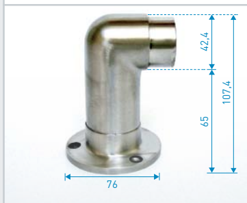
Seitenplatte 65 mm Nr. 100 • 42,4 mm • € 23,30
