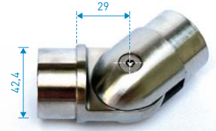
Gelenkstück Rohr/Rohr f. Rohr Nr. 250 • 42,4 mm • € 26,10
